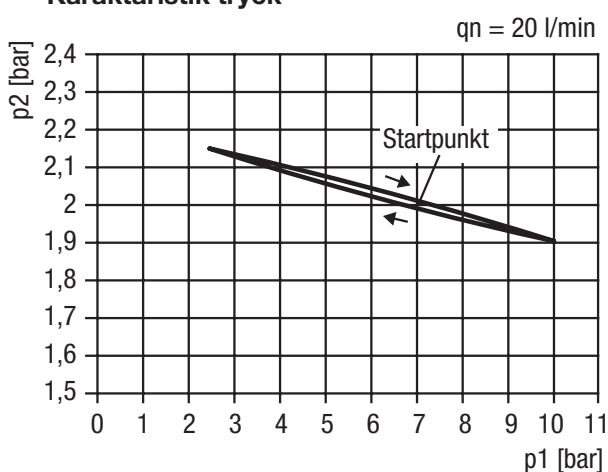
Karaktäristik tryck
