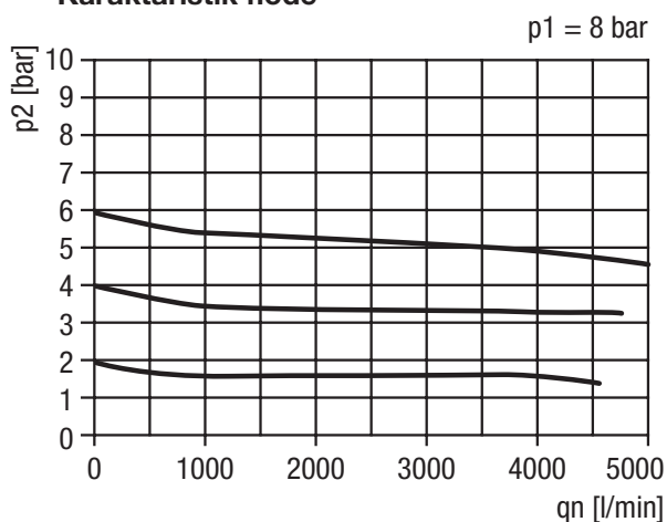
Karaktäristik flöde
